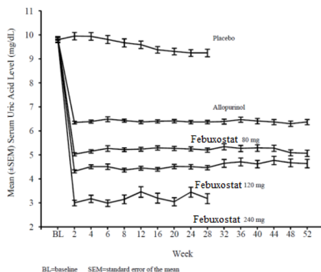
Figur 1: Genomsnittliga urinsyranivåer i serum i kombinerade pivotala fas 3-studier
