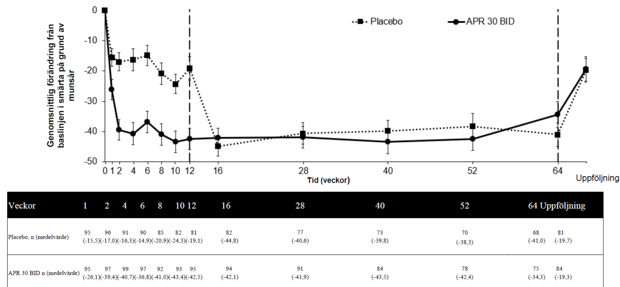
Figur 4. Genomsnittlig förändring från baslinjen i smärta på grund av munsår på en visuell analog skala enligt tidpunkt till och med vecka 64 (ITT-population; DAO)
