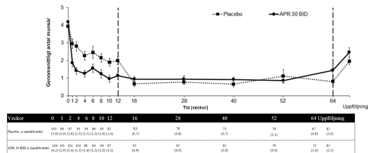
Figur 3. Genomsnittligt antal munsår enligt tidpunkt till och med vecka 64 (ITT-population; DAO)
